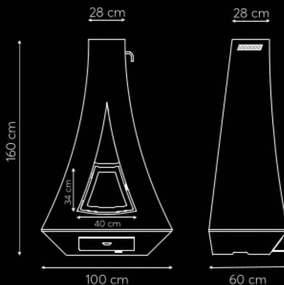
OUVERTURE LATÉRALE POUR SIMPLIFIER LE NETTOYAGE
